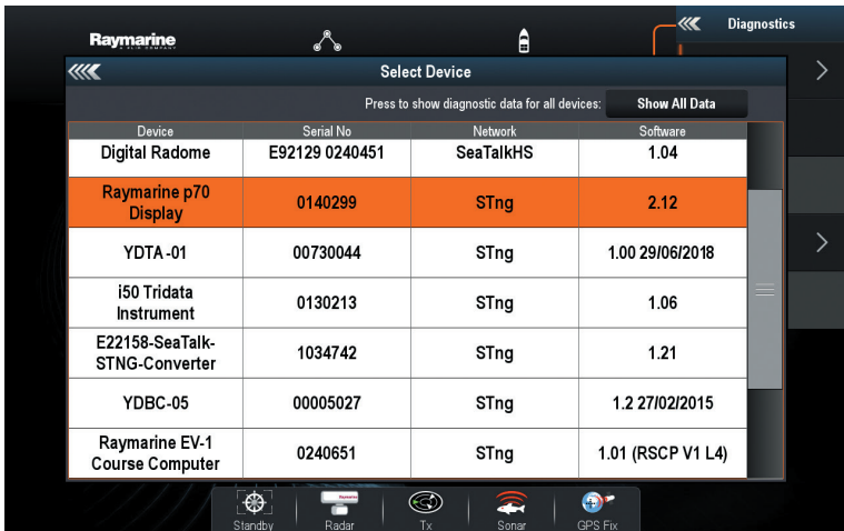
Figure 7. Raymarine c125 MFD «Device List» showing YDTA-01 unit.
